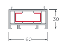
Utiliza ref. marco corredera 1.2mm - TC Perfil Elevación S60 30mm
