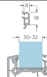
con junquillo 20-22 Sliding Acristalamiento 30-32mm
