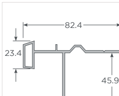
Utiliza ref. hoja corredera 98 / 2mm - TC Perfil Elevación S60 60mm
