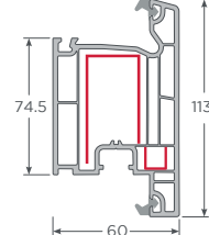
Con Ref. bisagra hoja puerta S60 1.2mm Hoja Puerta Exterior
