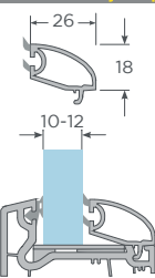
con junquillo 4-5 Sliding Acristalamiento 10-12mm
