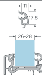
con junquillo 17-20 Sliding Acristalamiento 26-28mm
