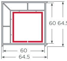
Esquinero 90° - 60mm S60
