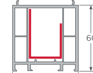
Utiliza ref. hoja corredera 98 / 2mm - TC Perfil Elevación S60 60mm
