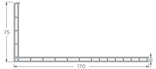
Ángulo de revestimiento 75 / 170mm
