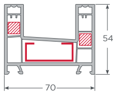
con Apoyo cerrado 9x9 - M Marco Doble Riel Corredera
