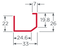
Ref. New Múltiple 2mm - TC PL-CMP-TC-MLT-2
