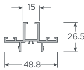
Adaptador Cuarta Hoja con Felpa
