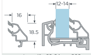
con junquillo 22-24mm S60 Acristalamiento 12-14mm
