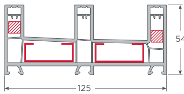
con Apoyo cerrado 9x9 - M Marco Triple Riel Corredera
