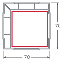
Esquinero 90° - 70mm Corredera
